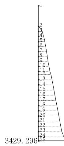
軸力(kN)
