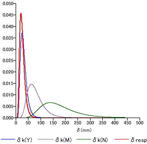
各損傷(C,Y,M,N)および応答(Resp)の確率密度関数(対数正規分布)
